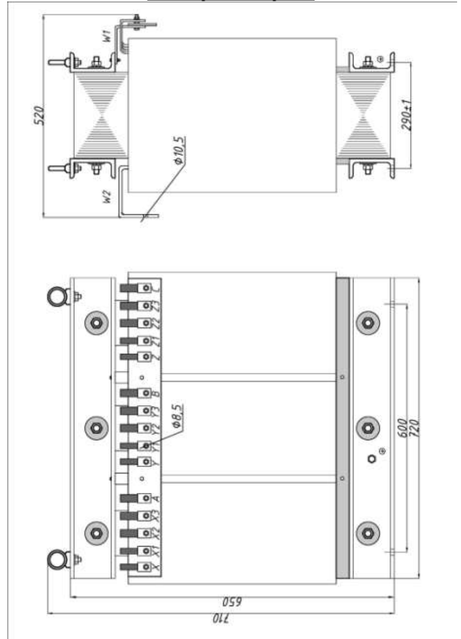
2.2 Габаритный чертеж
