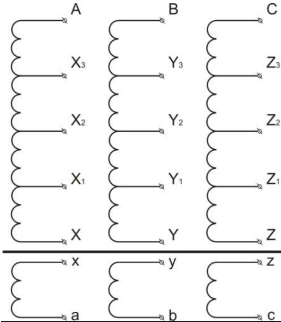
2.1 Схема электрическая принципиальная
